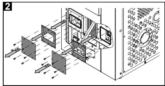
Rysunek 3c: Demontaż ściany bocznej (HSP 6 Rueda C PGI)
