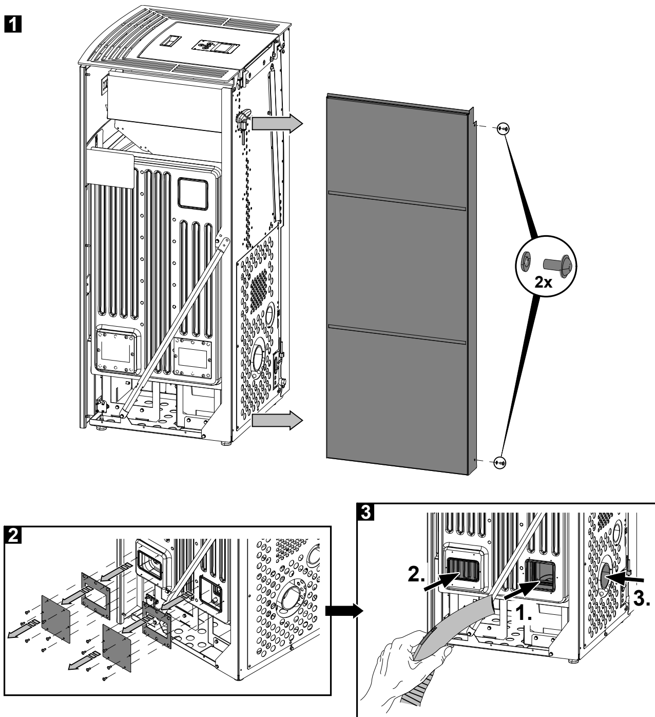
Rysunek 3a: Demontaż ściany bocznej (HSP 6 Rueda PGI)
