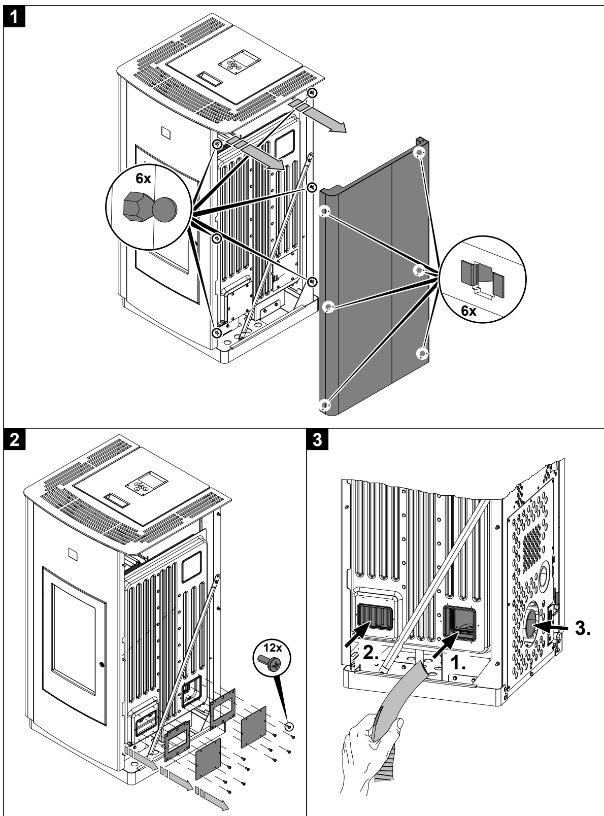
Rysunek 3b: Demontaż ściany bocznej
