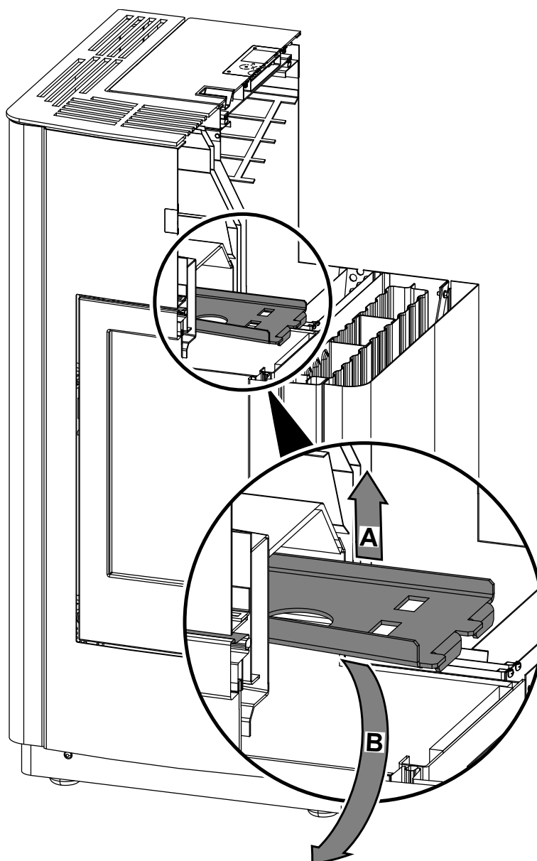
Rysunek 3a: Demontaż okładziny ciągu
